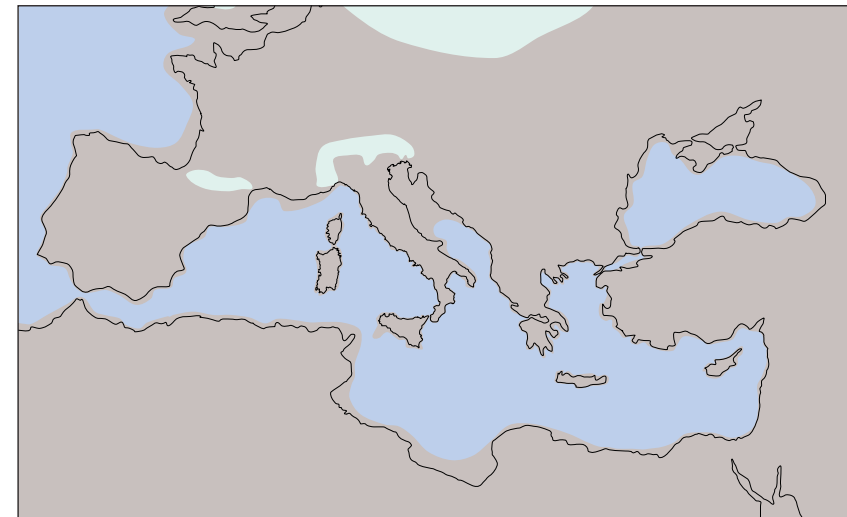
Paleogeografia semplificata del Mediterraneo nel Würmiano; marrone: aree emerse, azzurro: bacini marini, verde: coltri glaciali più estese
